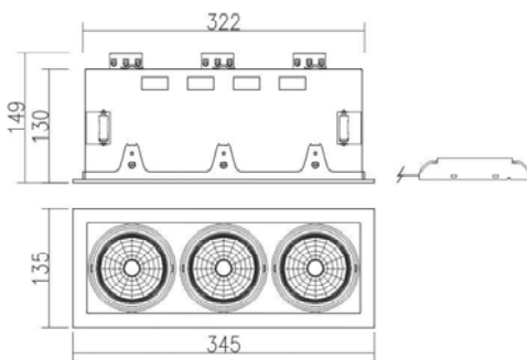
Technische Zeichnung
